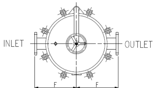
Eye bolt closure with hinge lid Augenschraubenausführung, Deckel klappbar
