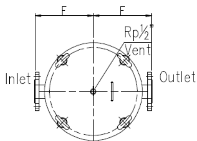
Clamp closure with hinge lid Spannklammerausführung, Deckel klappbar
